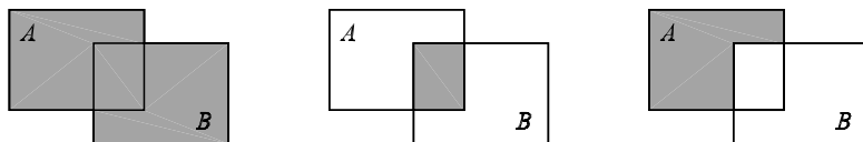
Sl. 1.1. Unija dvaju skupova (lijevo), presjek (u sredini) i razlika (desno).
